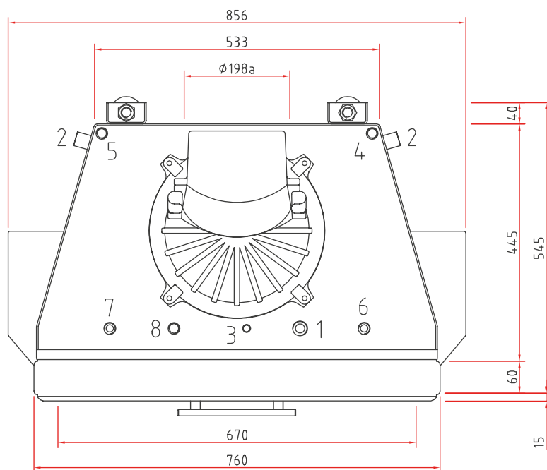
Widok z góry, skala 1:10
