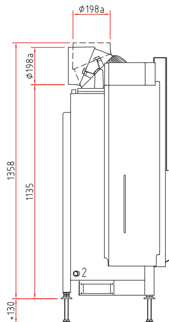
Widok z boku, skala 1:20
